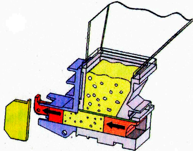
Messkammer füllen Füllvorgang beginnt erst, wenn Messer vollständig geschlossen
