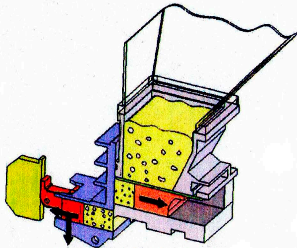
Haupt-u. Messkammer entspannen Komprimierte Gase können sich bei geschlossenem Messer wieder entspannen. Kein zerquetschen des Teiges, keine Pumpenbewegung im Trichter.
